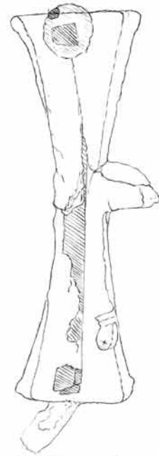
Eiserne Klammer mit Bleiverguß in Schwalbenschwanz-Bettung
