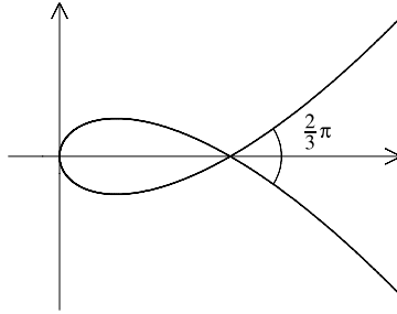
Fig. 2. Tschirnhausen cubic
