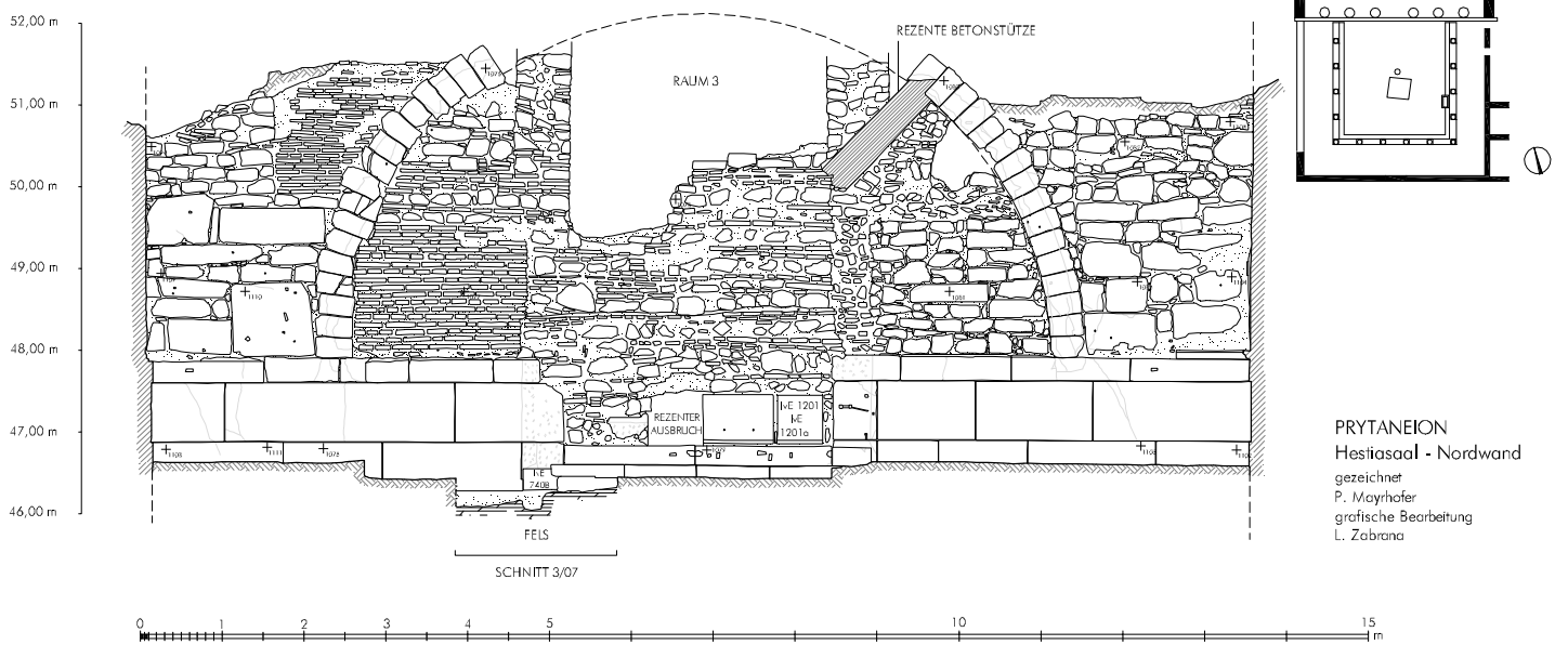
2 ›Hestiasaal. Nordwand (1:100)
