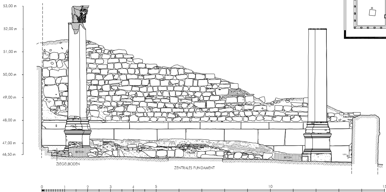
2 ›Hestiaaal‹. Nord-Süd-Schnitt nach Osten (1:100)
