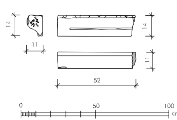
PRYTANEION HESTIASAAL - PR 33/03 B GESIMS-FRAGMENT gezeichnet N. High grafische Bearbeitung L. Zabranca
