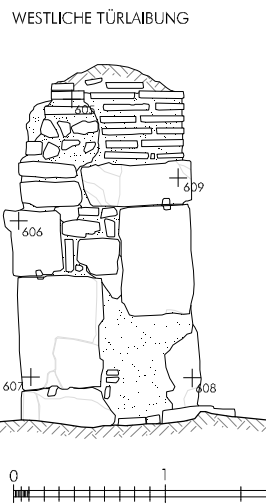
4 ›Hestiasaal‹. Westliche und östliche Türlaibung von Tür 3 (1:50)
