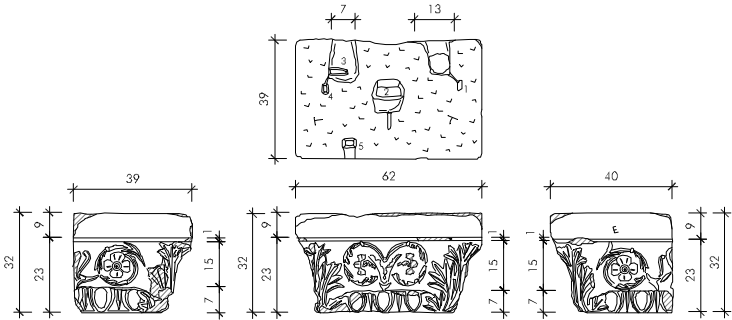
3 Pilasterkapitell A 45
