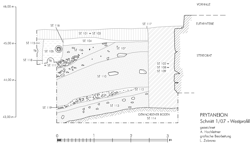
1 Schnitt 1/07. Westprofil (1:50)
