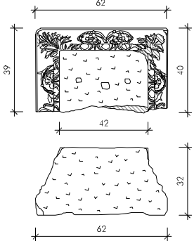
4 Pilasterkapitell A 45 (1:25)
