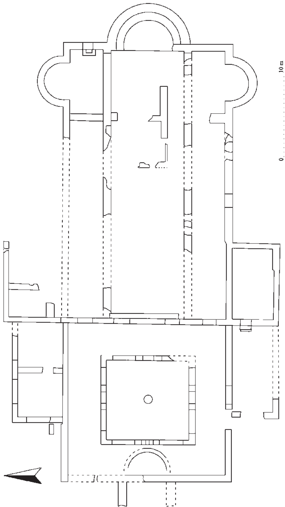
Abb. 9: Grundriss der Basilika von Arapaj
