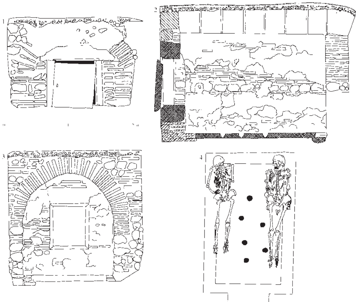
Abb. 19/1–4: Grabkammer, Ansicht des Eingangs an der Ostseite, Ost-West-Schnitt durch die Kammer, Innenansicht der Ostwand mit dem Eingang
