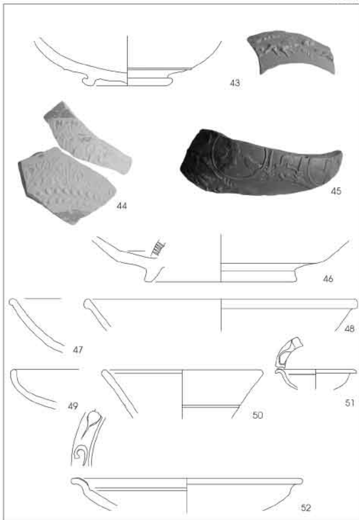
Feldkirchen: 43–52 Keramik M 1:2.
