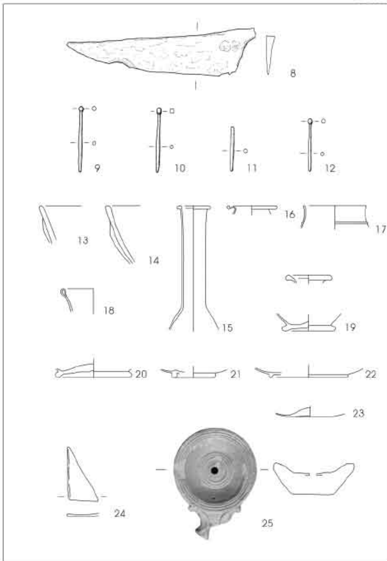
Feldkirchen: 8 Eisen; 9–12 Bein; 13–24 Glas; 25 Keramik M 1:3.
