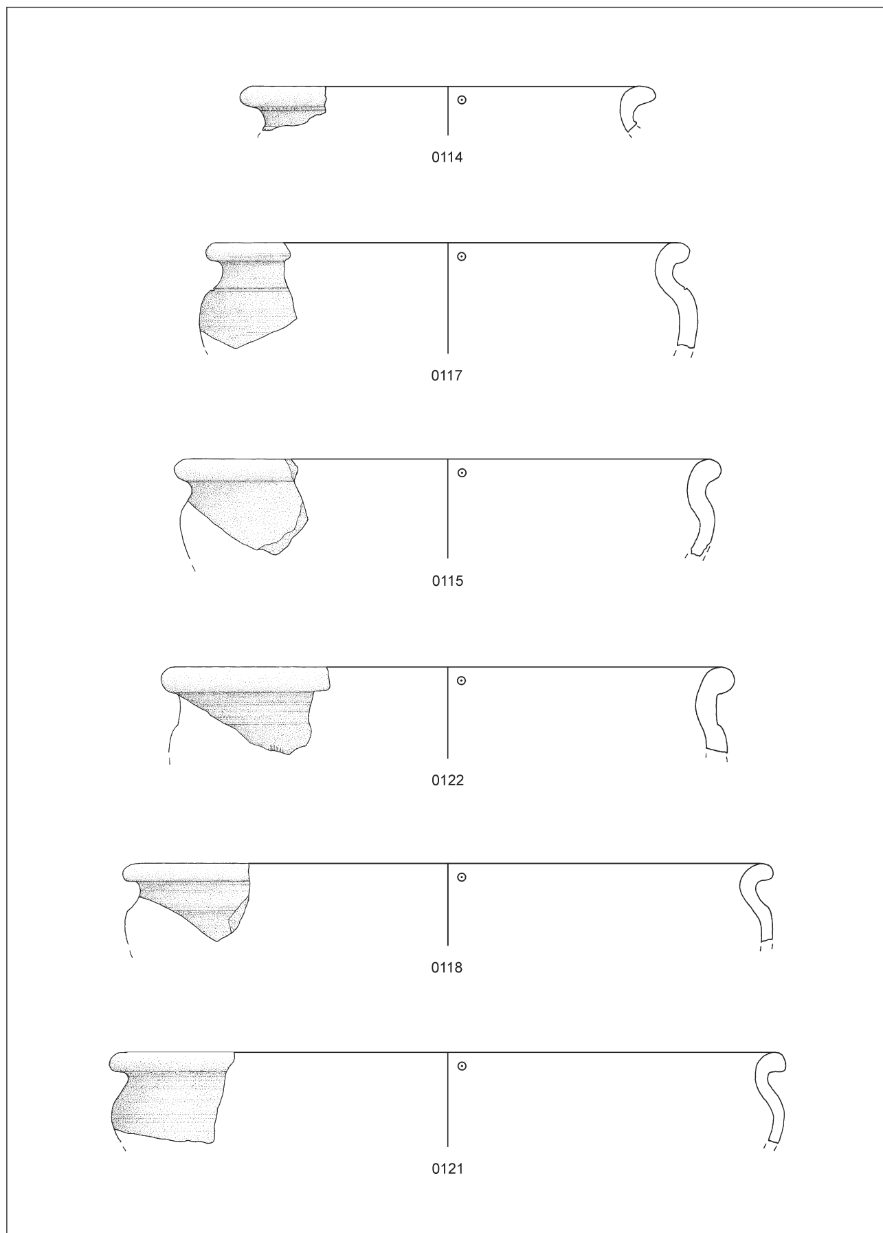
Tafel 18: Töpfe mit Mündungen der Form E1. M. 1:2.
