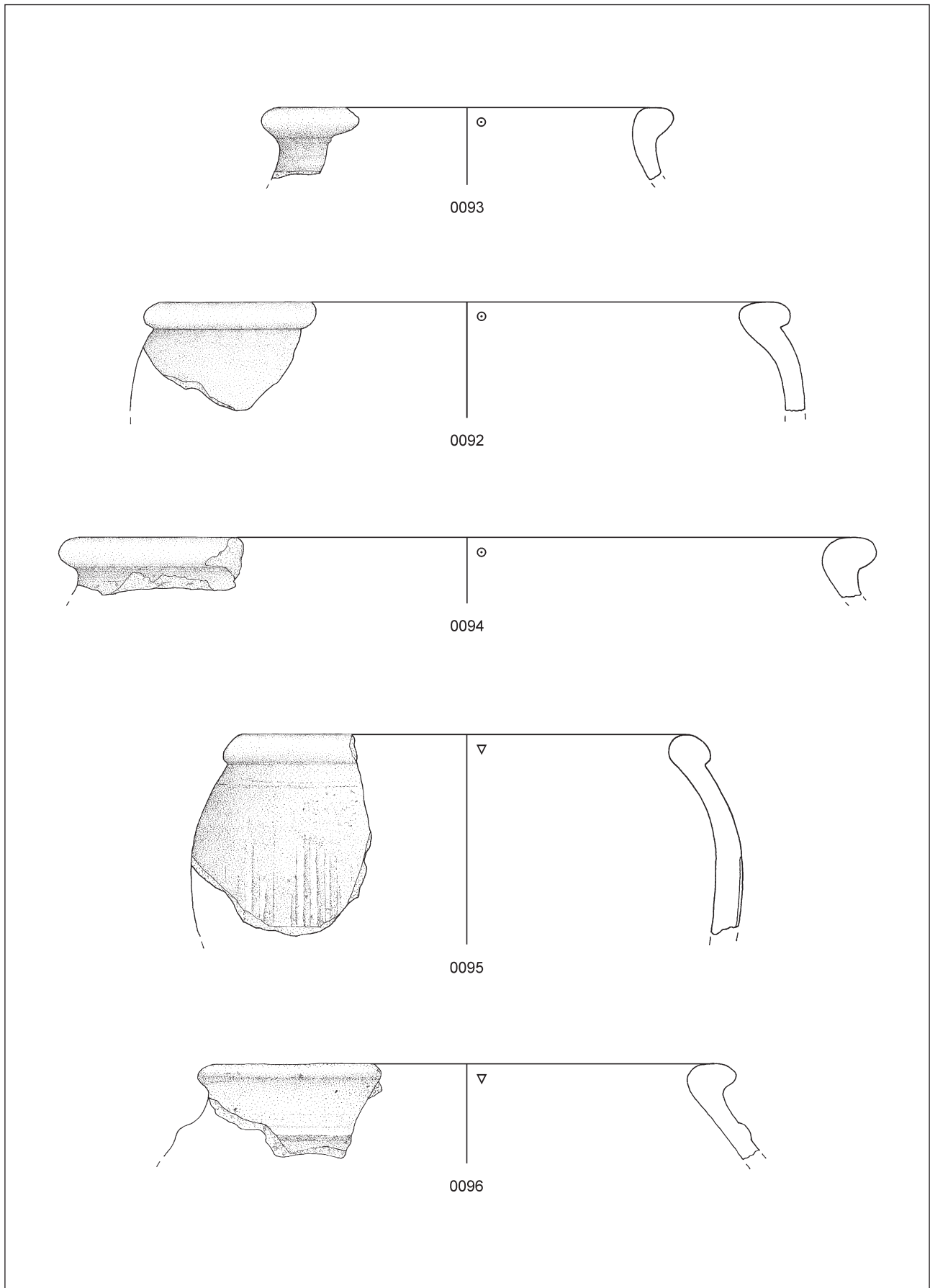
Tafel 15: Töpfe mit Mündungen der Form D1. M. 1:2.
