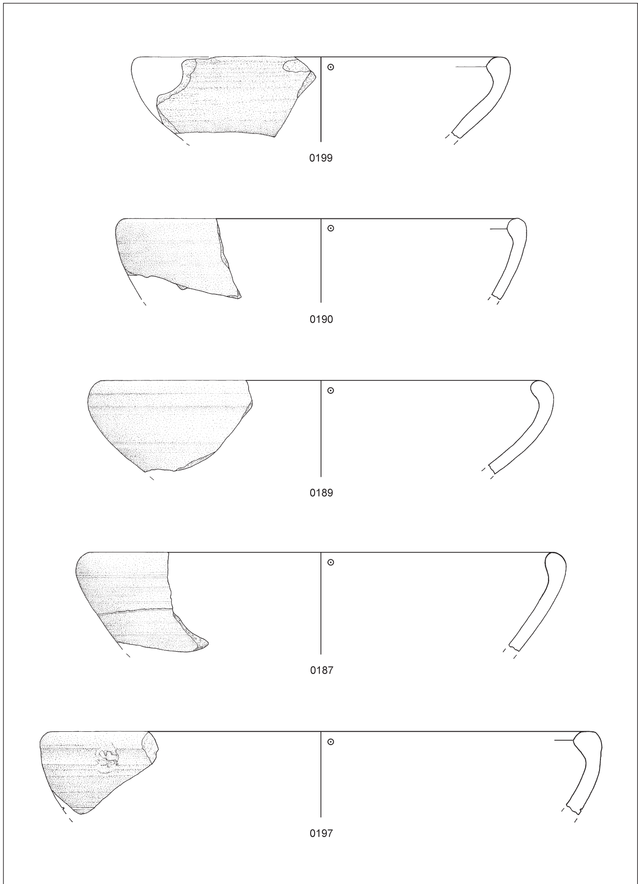
Tafel 25: Schüsseln mit Mündungen der Form K1. M. 1:2.
