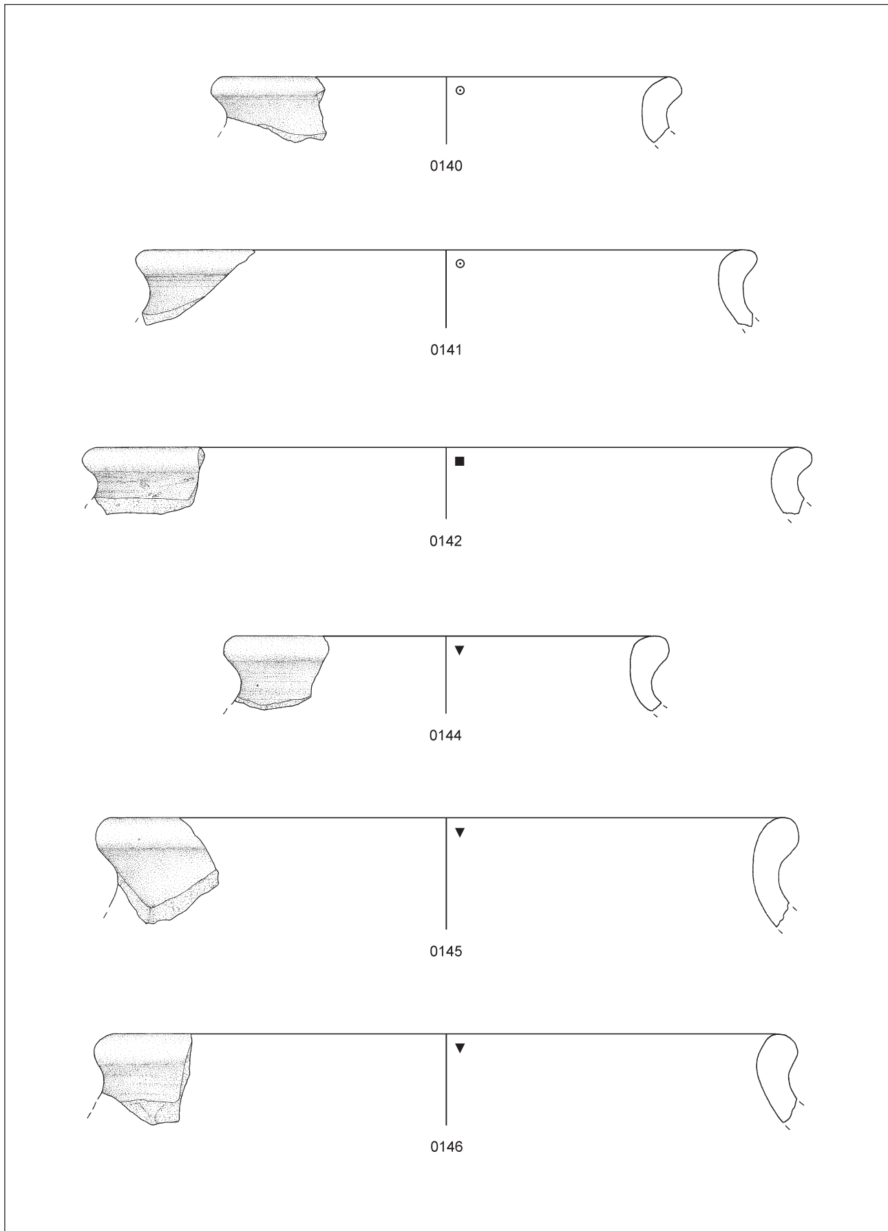
Tafel 21: Töpfe mit Mündungen der Form F. M. 1:2.
