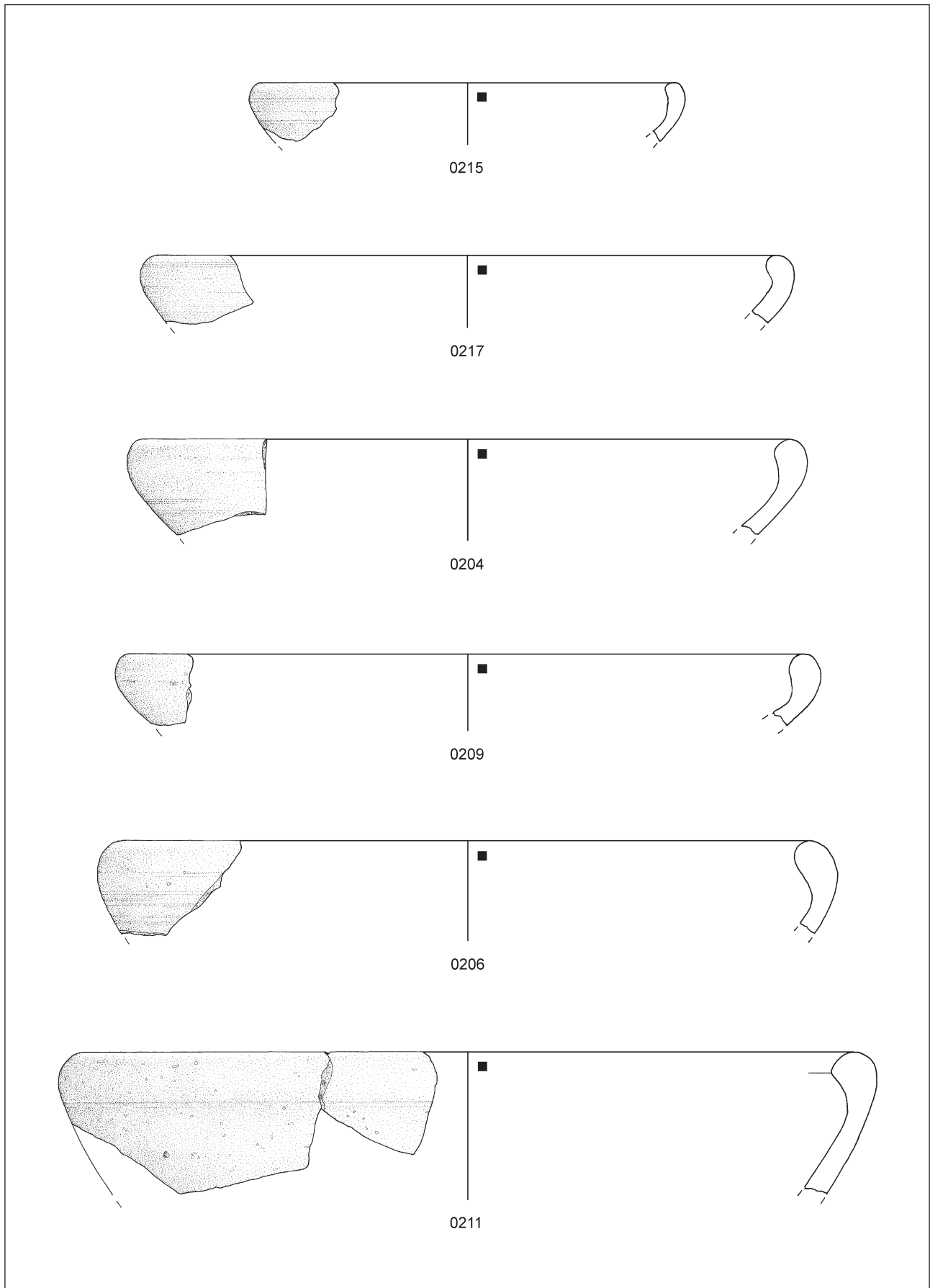
Tafel 29: Schüsseln mit Mündungen der Form K1. M. 1:2.
