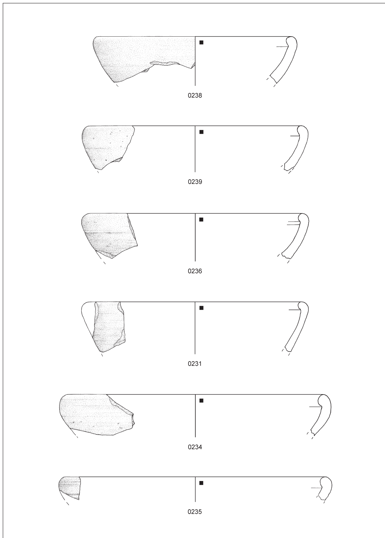
Tafel 33: Schüsseln mit Mündungen der Form K2. M. 1:2.
