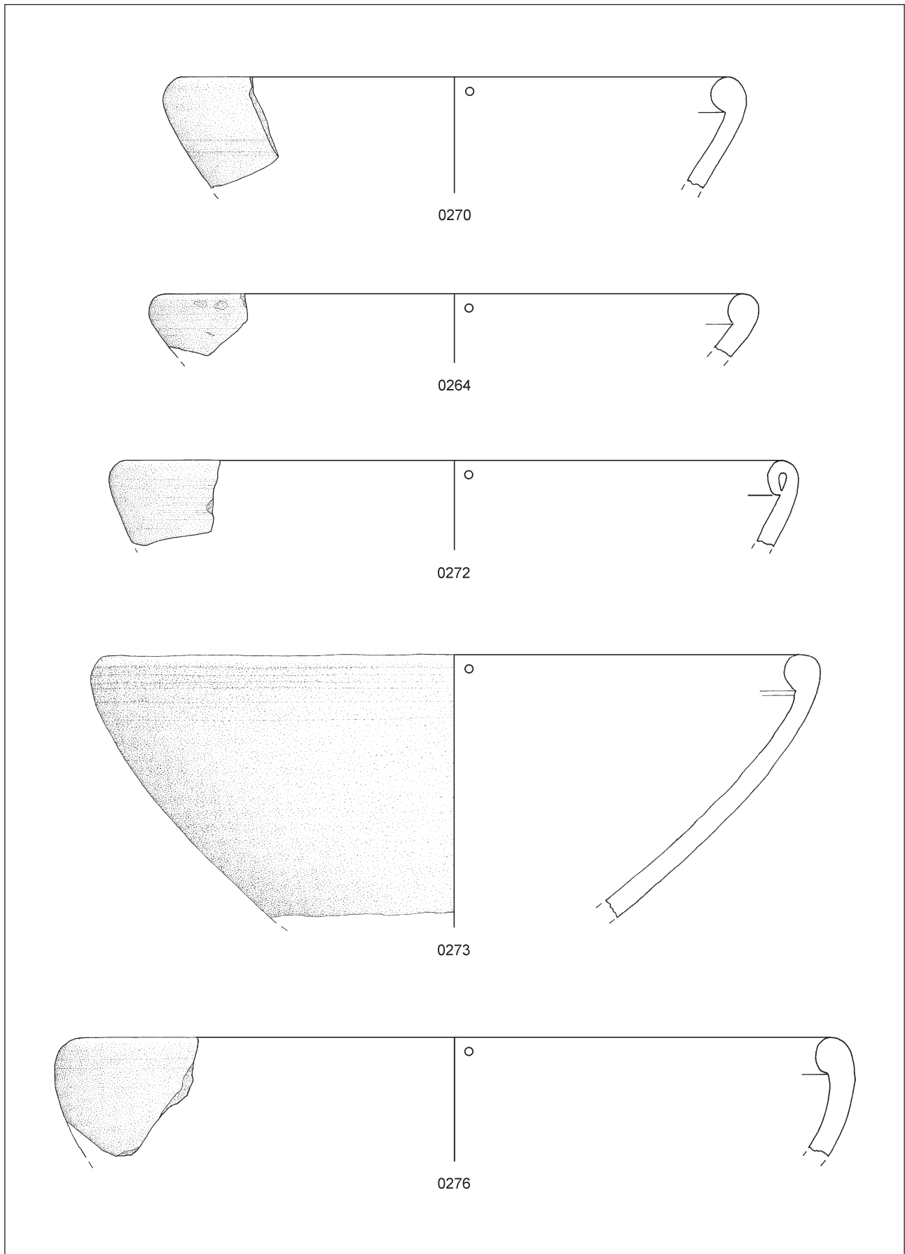
Tafel 37: Schüsseln mit Mündungen der Form L1. M. 1:2.
