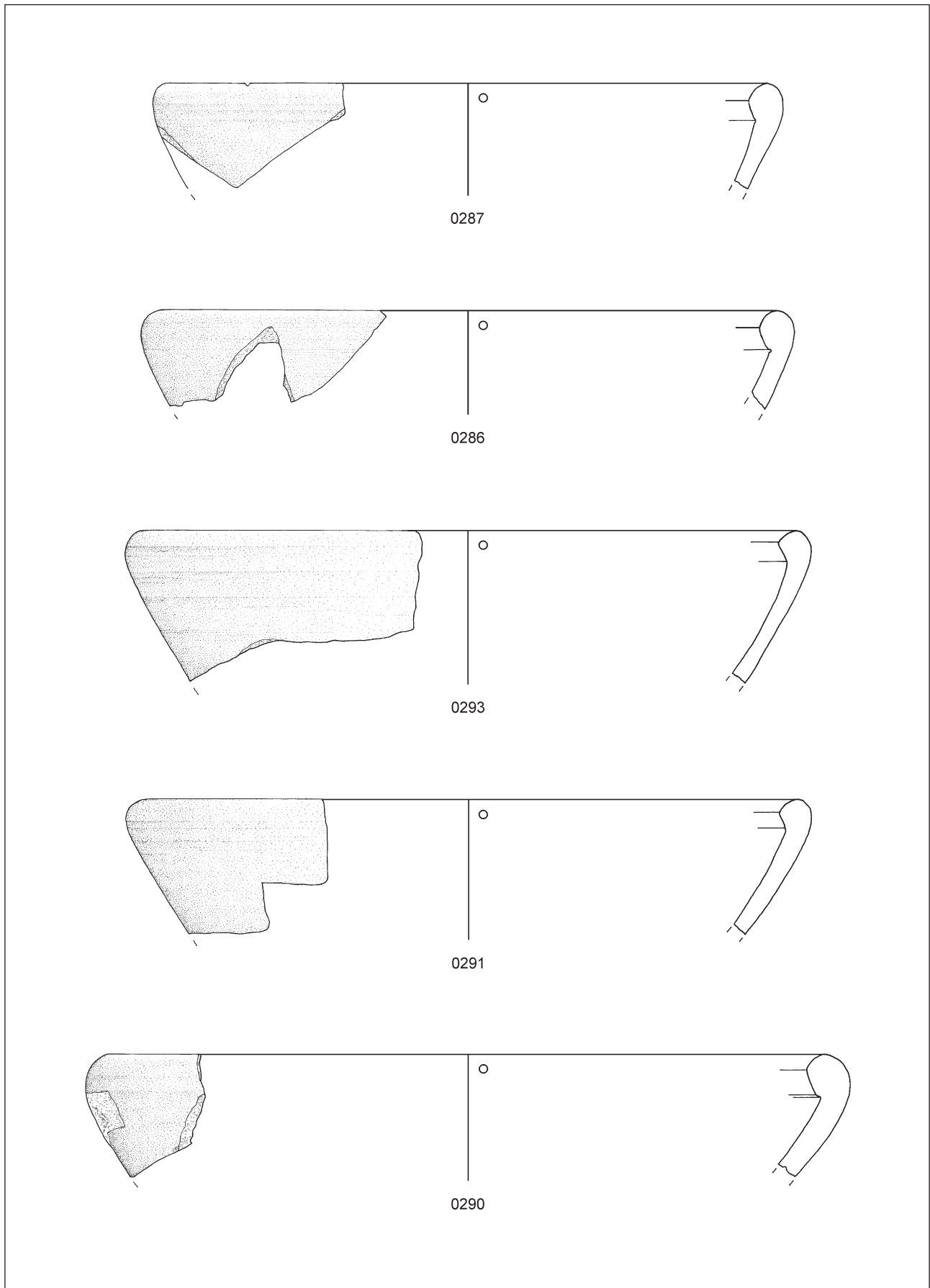
Tafel 39: Schüsseln mit Mündungen der Form L2. M. 1:2.
