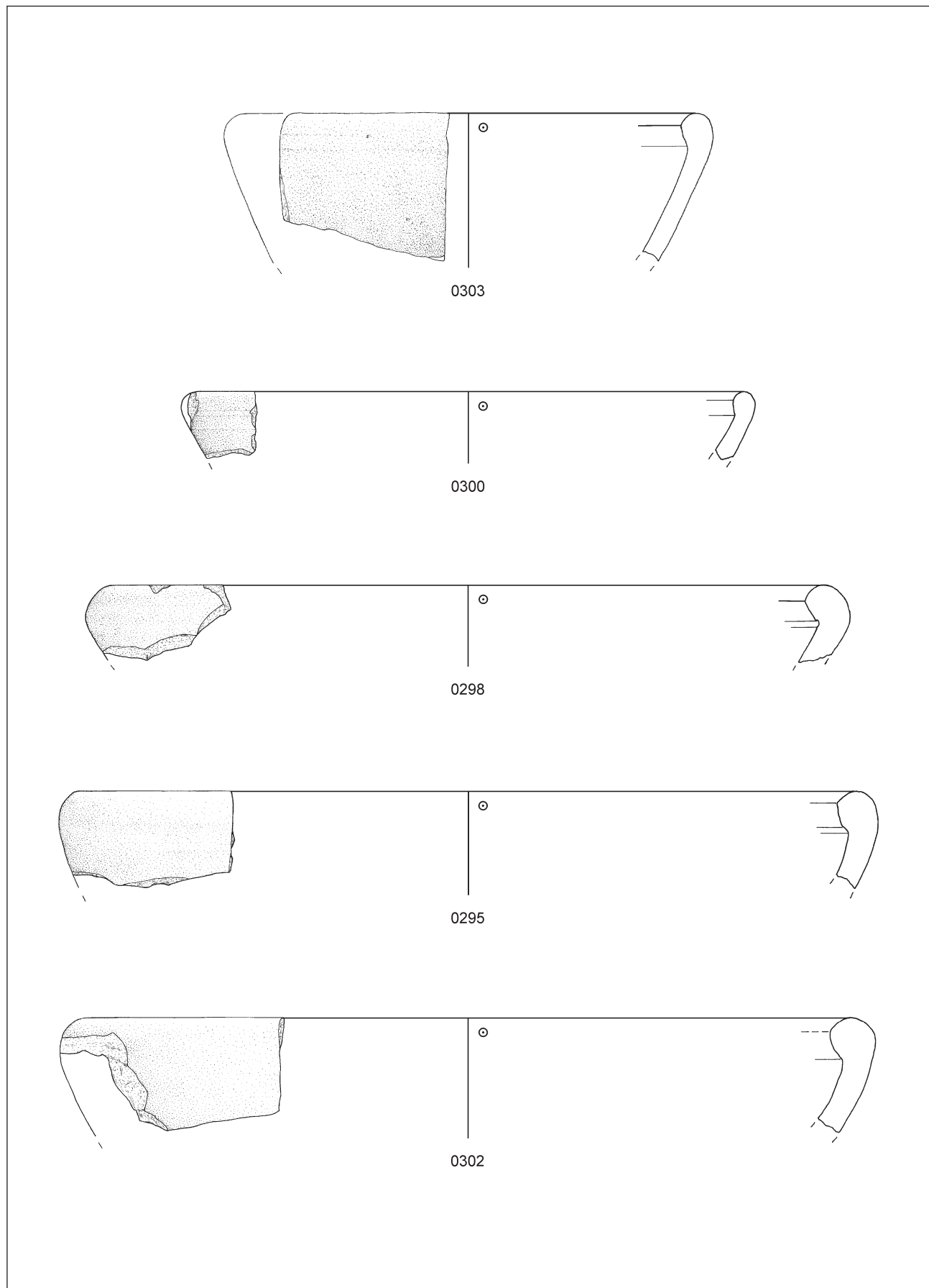
Tafel 41: Schüsseln mit Mündungen der Form L2. M. 1:2.
