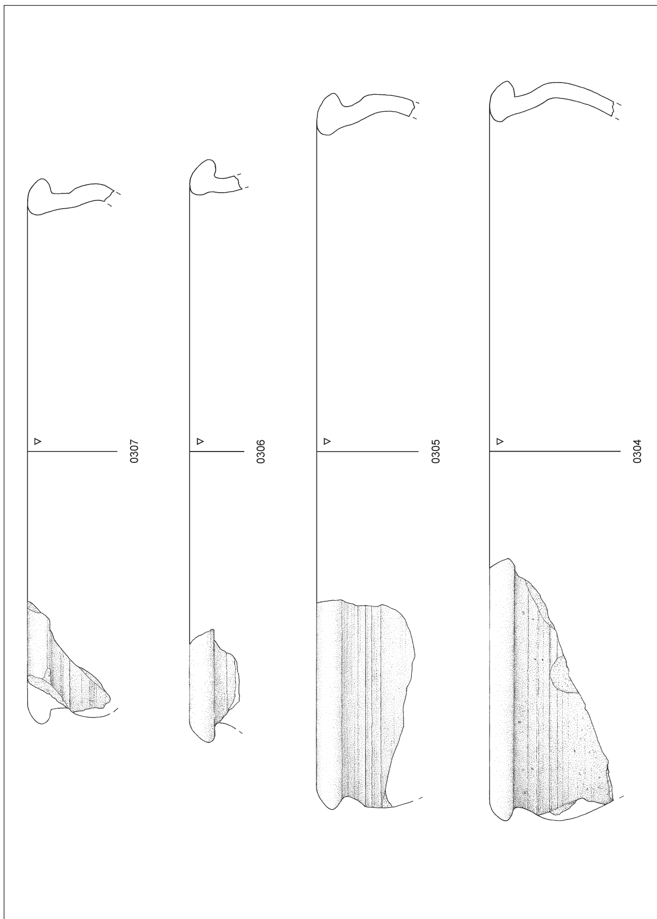
Tafel 42: Schalen mit Mündungen der Form M. M. 1:2.
