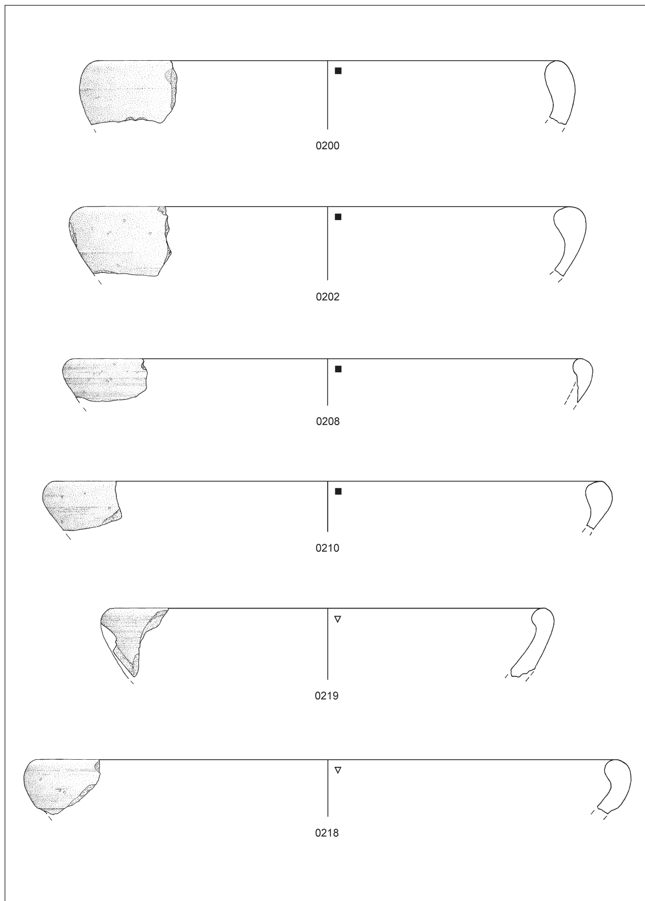
Tafel 30: Schüsseln mit Mündungen der Form K1. M. 1:2.
