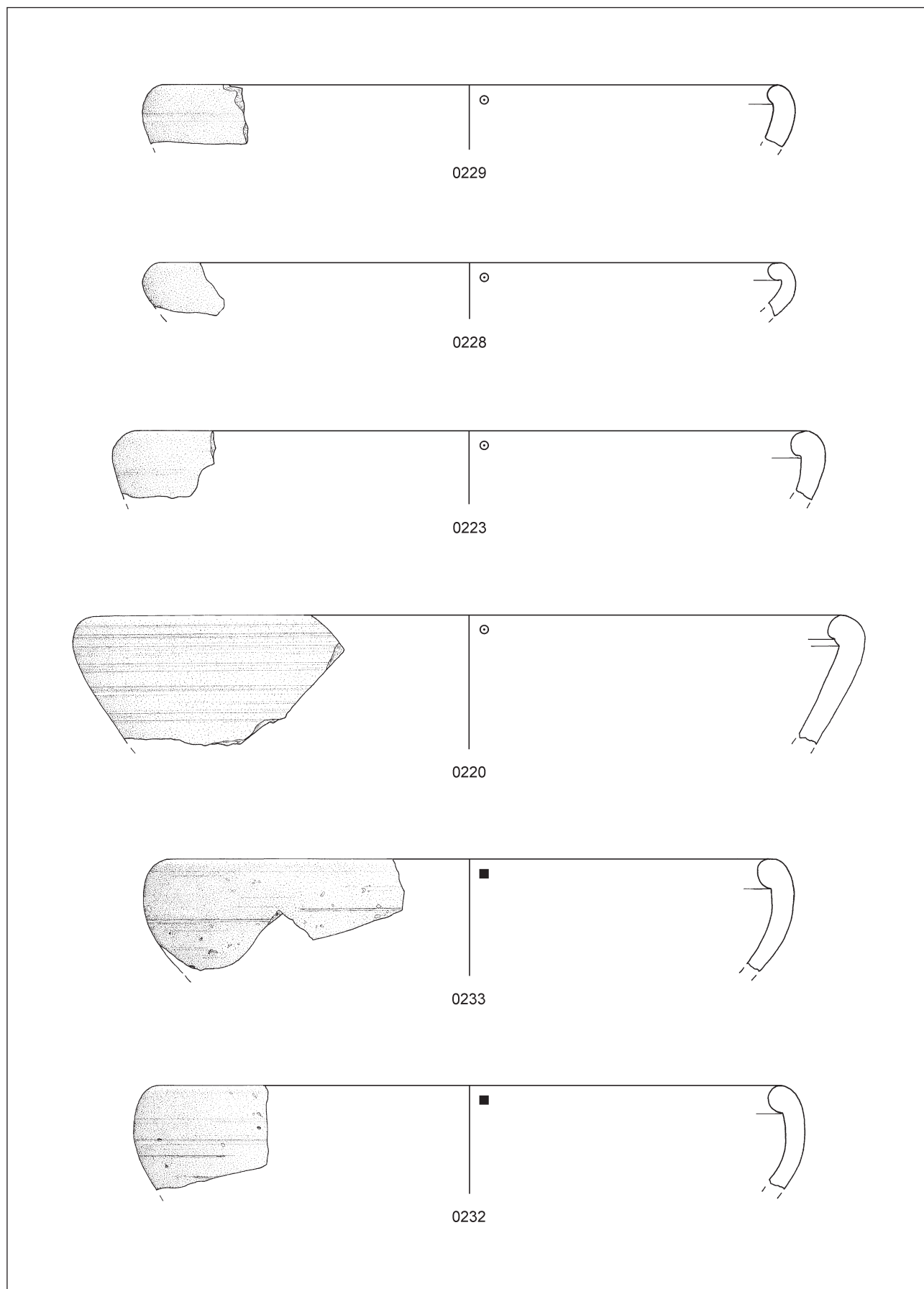
Tafel 32: Schüsseln mit Mündungen der Form K2. M. 1:2.
