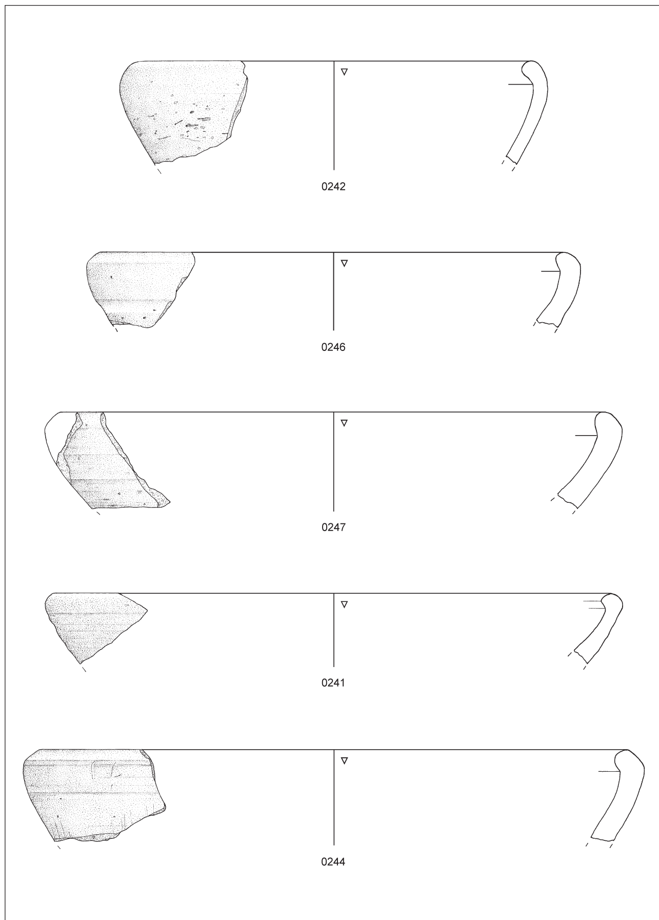
Tafel 34: Schüsseln mit Mündungen der Form K2. M. 1:2.
