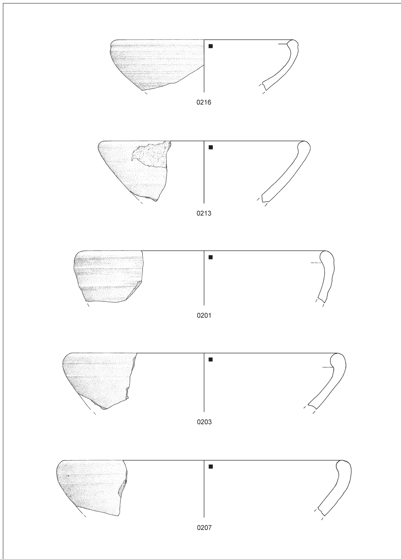
Tafel 28: Schüsseln mit Mündungen der Form K1. M. 1:2.
