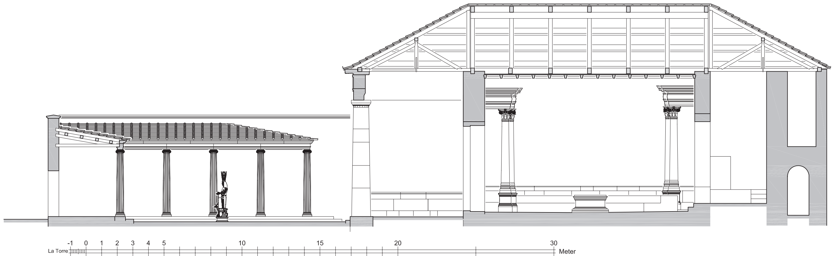
2 Prytaneion. Schnitt b-b' (1:150)
