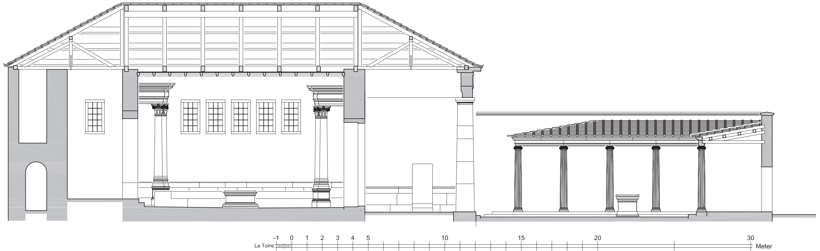
1 Prytaneion. Schnitt a-a' (1:150)
