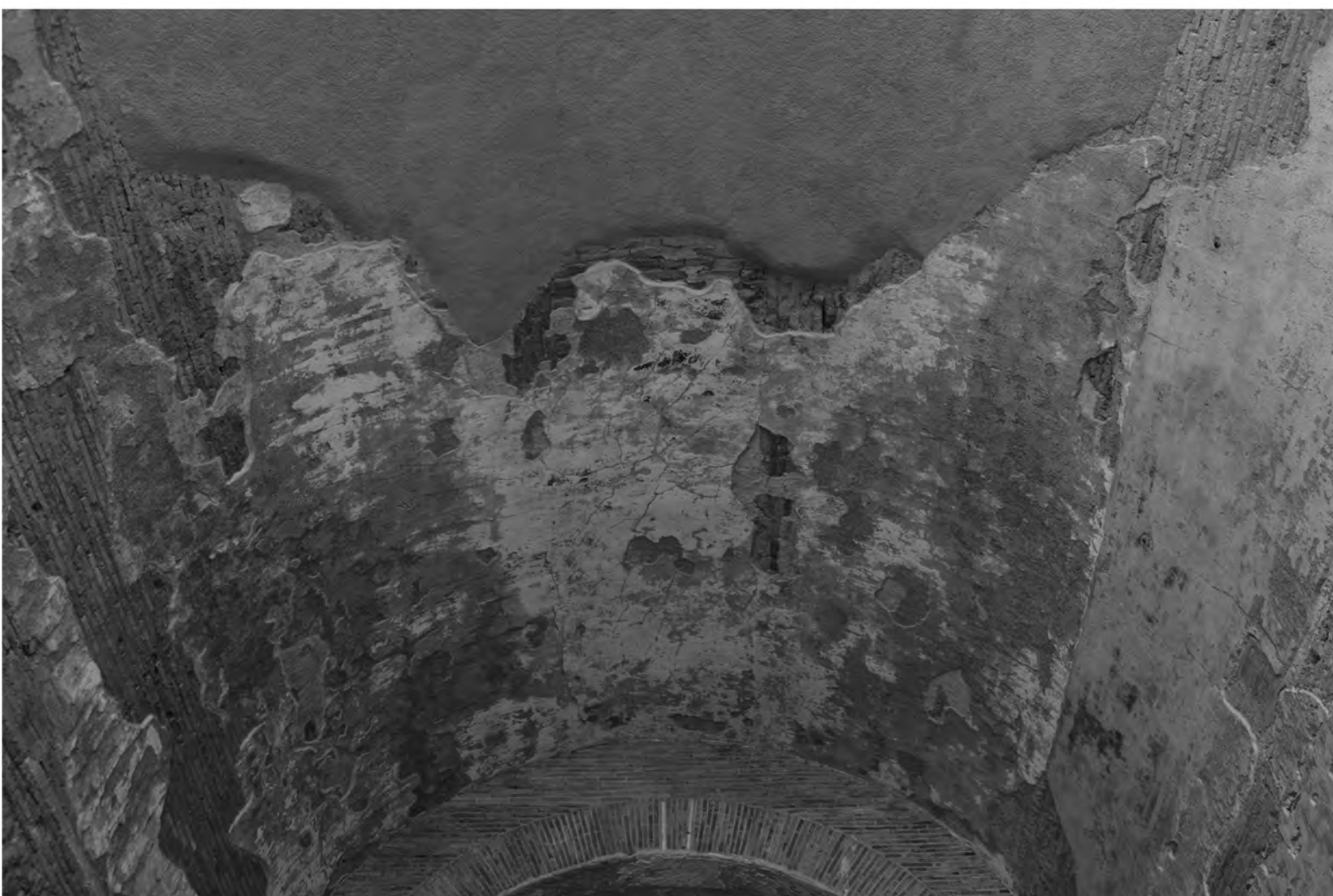
Abb. 26: Apsidensaal 8, Tonnengewölbe
