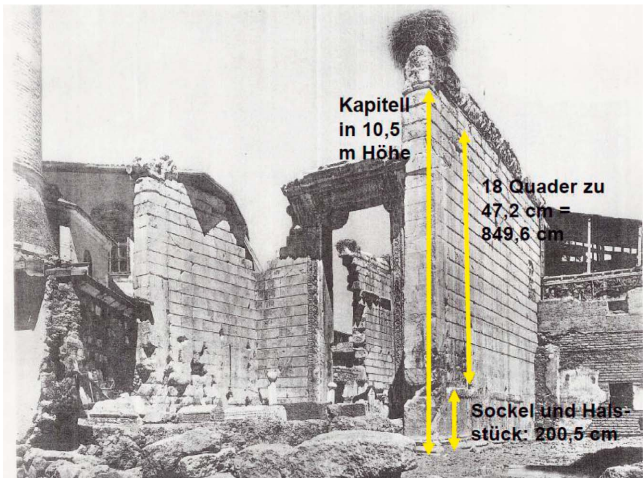
Abb. 5: Bemaßung der südlichen Cellawand (nach: KRENCKER – SCHEDE 1936, Taf. 13, Ergänzungen A. COŞKUN)
