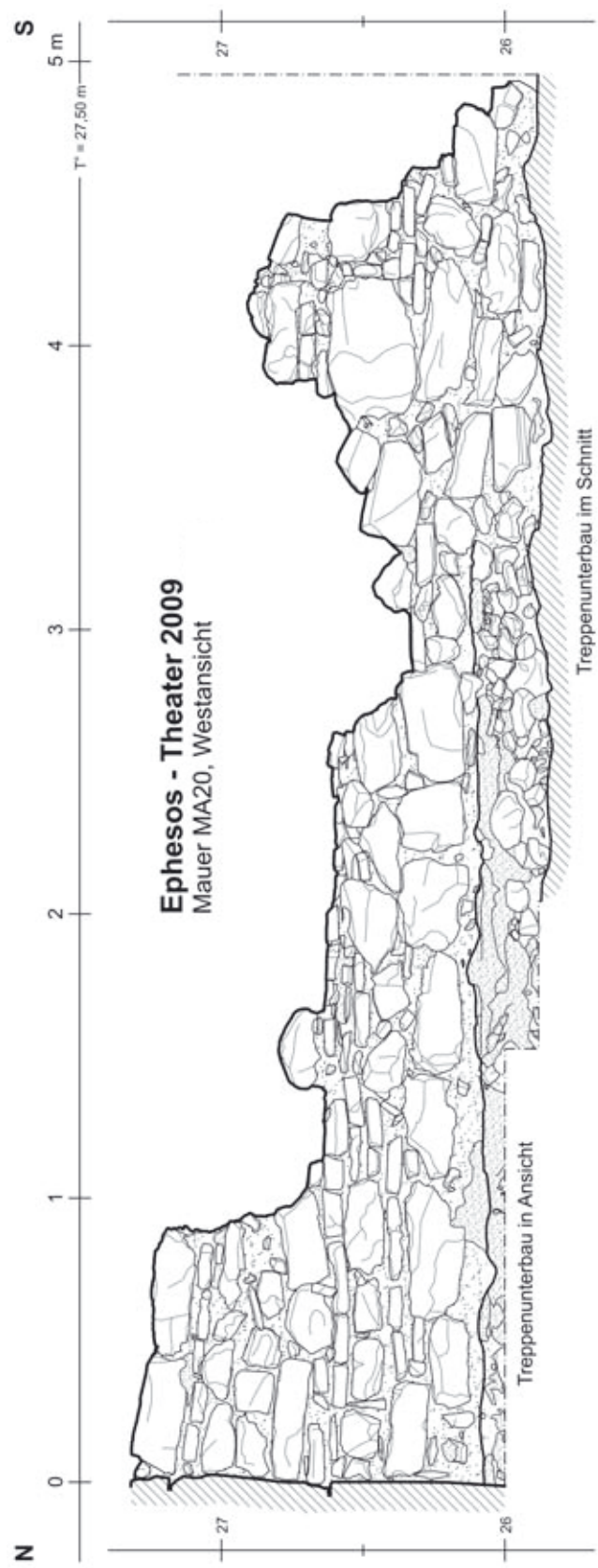
Abb. 540: MA20, W-Ansicht
