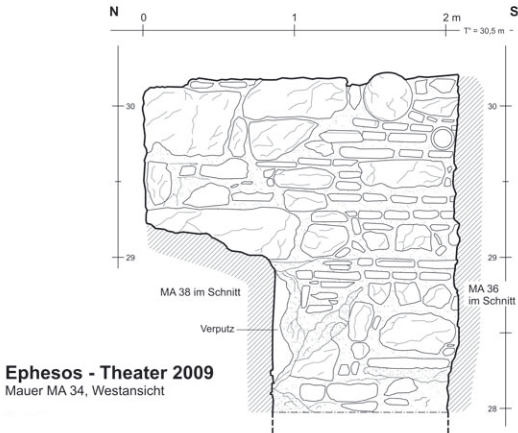
Abb. 518: MA34, W-Ansicht
