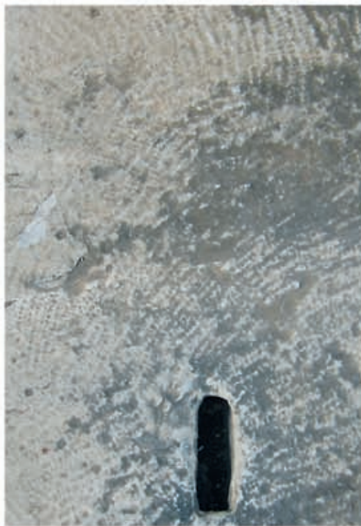
2 Grob gezahnte Lagerfuge des Architravs 100A (Draufsicht)
