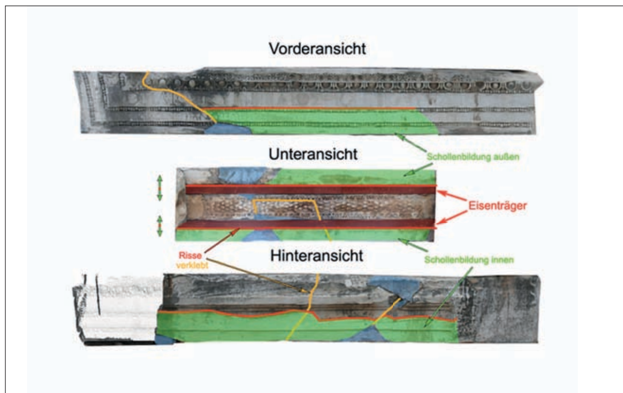
2 Akute Schäden an Block 040A
