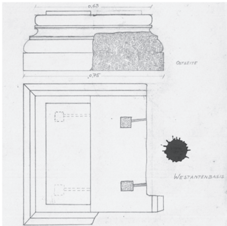
2 Pfeilerbasis 012B (Zeichnung K. H. Göschl)
