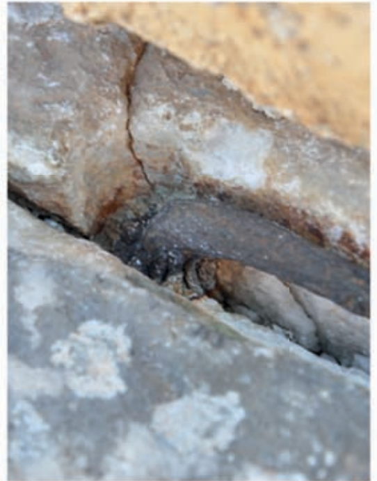
2 Eisenklammer zwischen 095L und 098D
