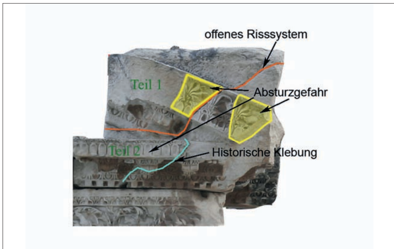
1 Akute Schäden an Block 053G
