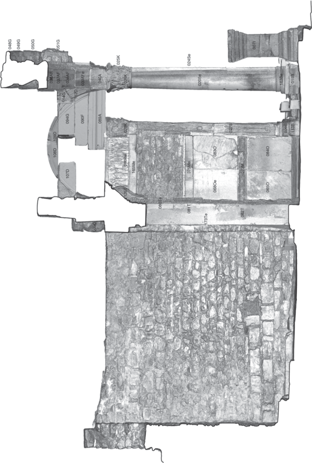
Rekonstruktion mit Bauteilkartierung Schnitt A-A'
