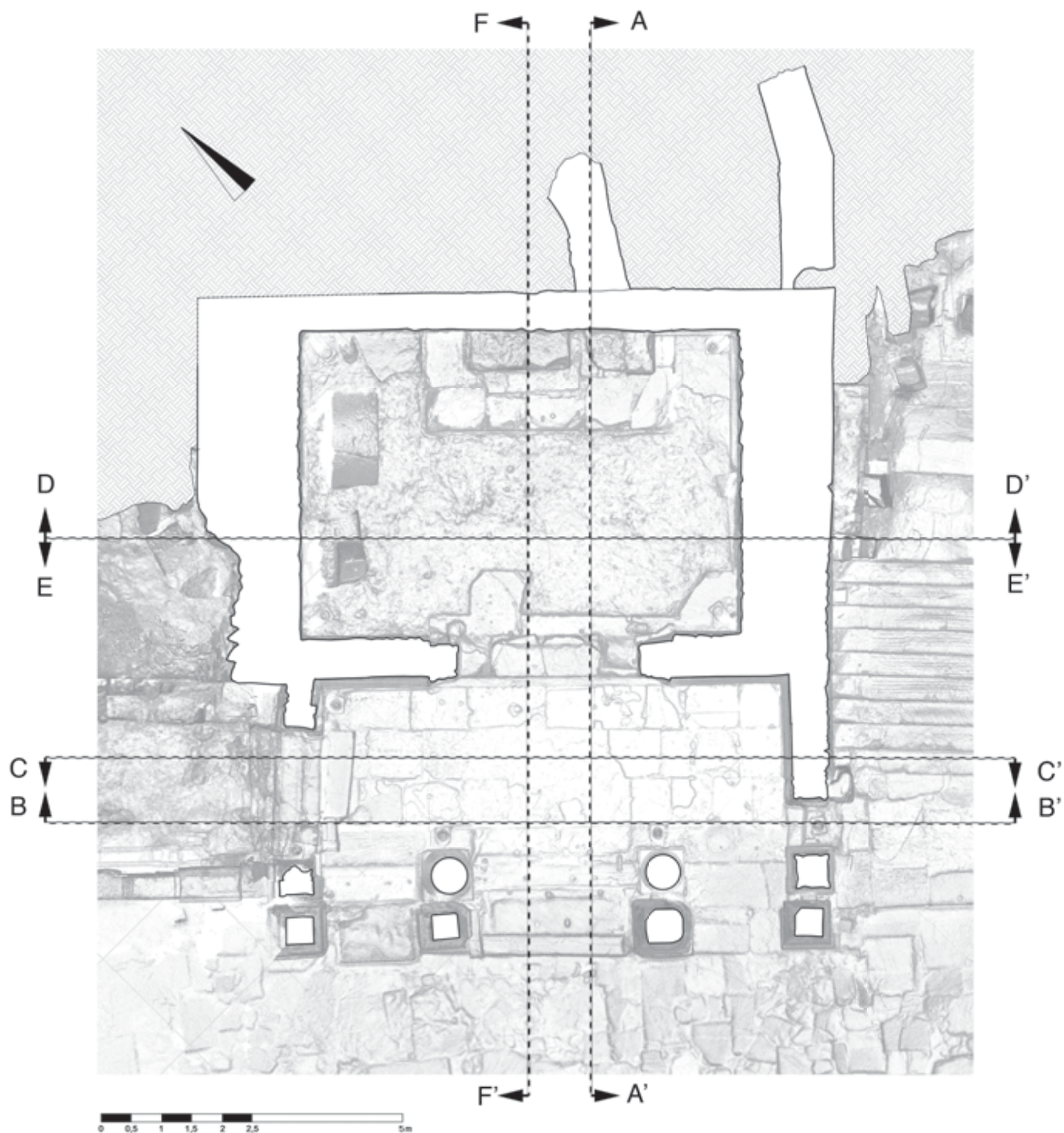
Grundriss mit Position der rekonstruierten Gebäudeschnitte (vgl. Taf. 203–209)
