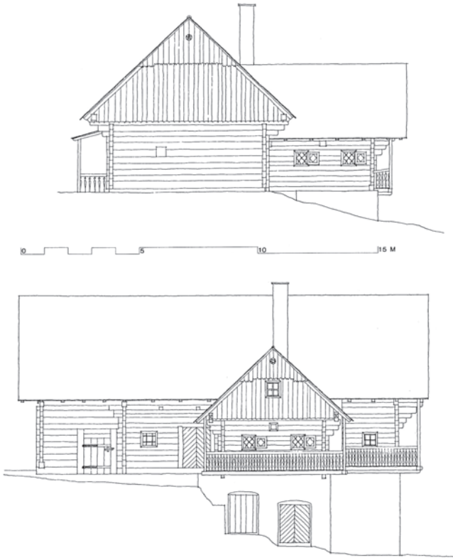
Abb. 5: Ligist, Dietenberg, Steiermark, Bauernhaus vulgo Leitnerhans, Bauaufnahme in „Steiermark – Alte Bauernhöfe“, 1992
