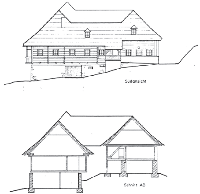
Abb. 6: Obdach, Steiermark, Bauernhof vulgo Schwarzhube, Bauaufnahme in „Das Umadumhaus“, 1979
