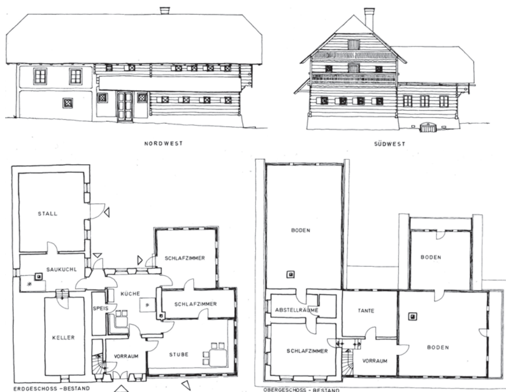
Abb. 4: Birkfeld, Steiermark, Bauernhaus vulgo Schirnhöfer, Planaufnahme für das Forschungs- und Sanierungsprojekt der Steiermärkischen Landesregierung, 1978
