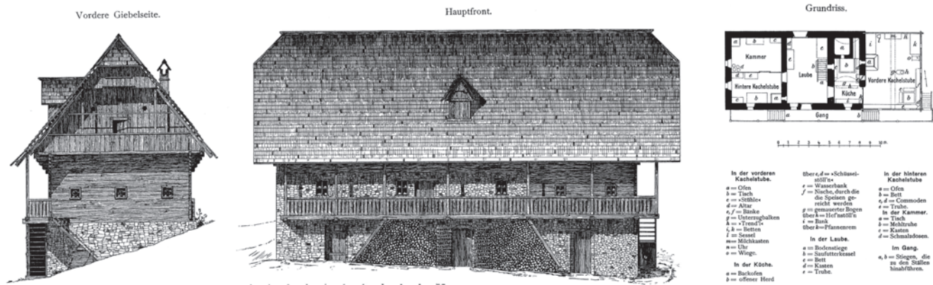
Abb. 1: Köflach, Steiermark, Bauernhaus vulgo Jud, Plandokumentation in „Das Bauernhaus in Österreich-Ungarn“
